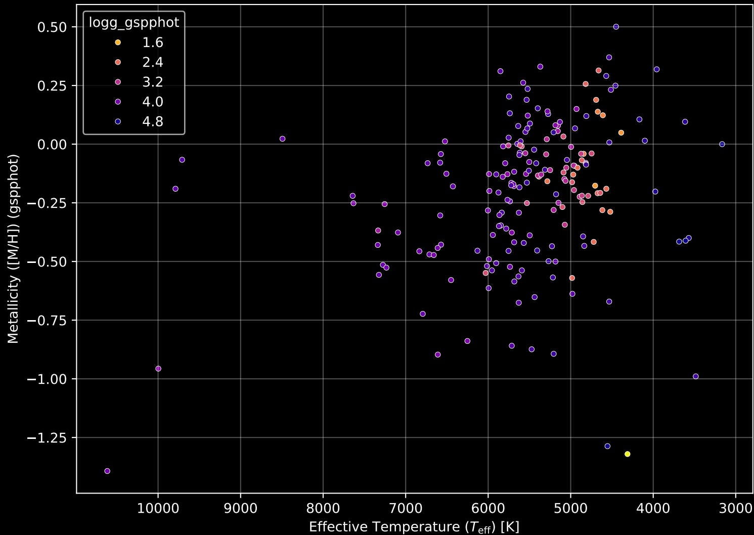
APOGEE DR17 Field: [085+35_MGA] Stellar Population Parameters (n= 193)
